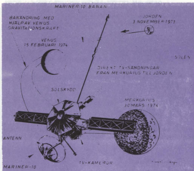
Så här rymdflög Mariner 10 från Jorden, förbi Venus och Merkurius.
